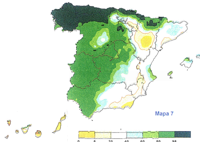
SITUACIÓN EMBALSES
