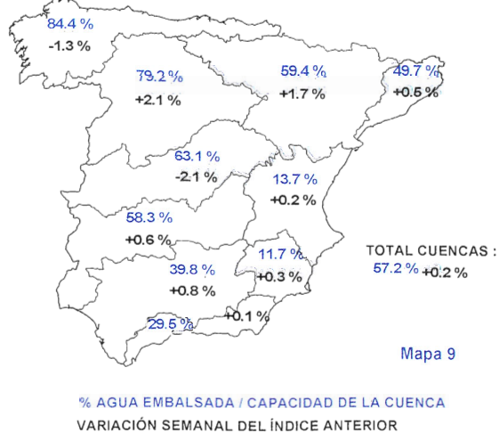
SITUACIÓN EMBALSES
