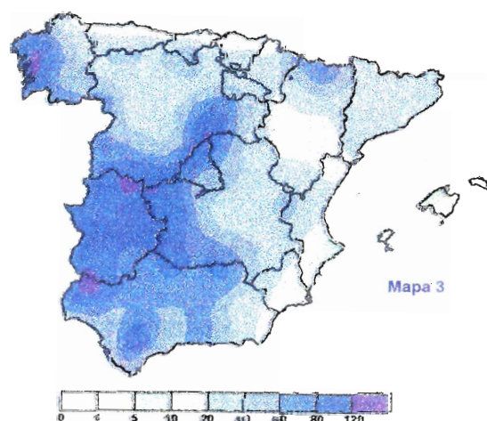
PRECIPITACIÓN ACUMULADA (mm) EN LA DÉCADA.
