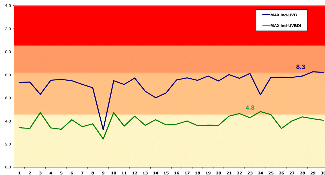
Evolución del Índice Máximo diario de Radiación UVB y UVB Difusa - MADRID ABRIL 2015
