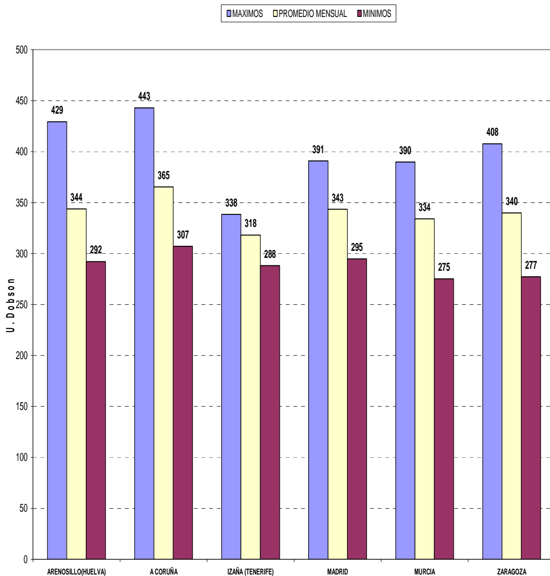
DATOS MENSUALES DE OZONO EN COLUMNA - ABRIL 2015
