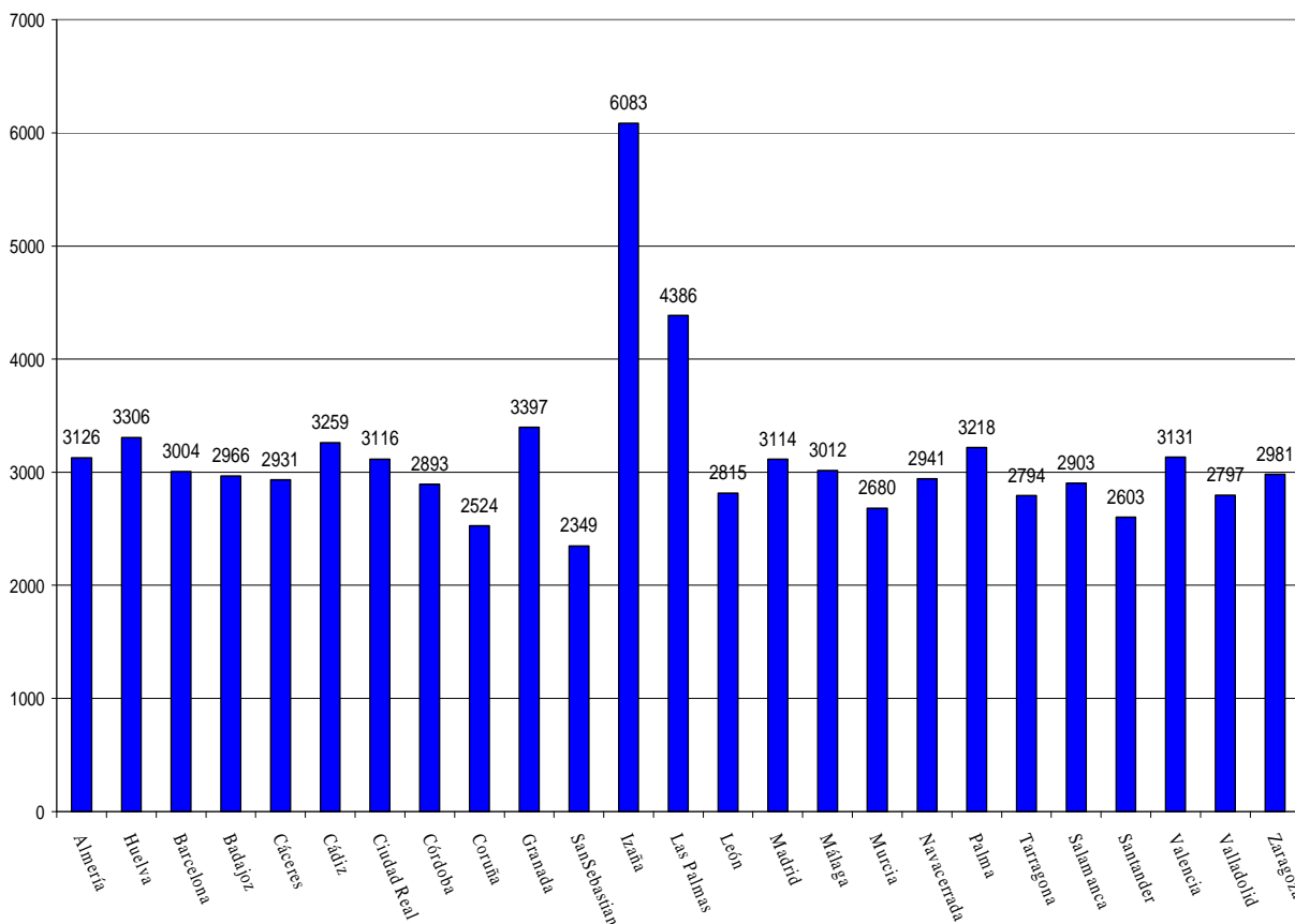
VALORES MEDIO DIARIOS DE LA RADIACIÓN UV-B EN DISTINTAS ESTACIONES DE LA RED ABRIL-2015 (J/m 2 )
