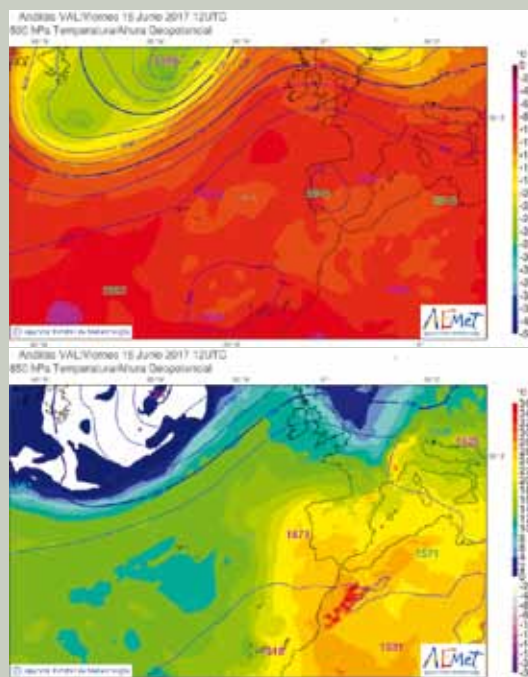
Fig. 1 y 2. Topografías de 500 y 850 hPa del 16 de junio
