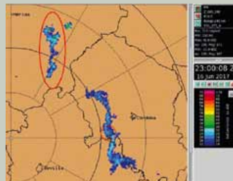
Figura 11. PPI del radar de Sevilla mostrando dos ecos en forma de serpiente o serpentina. En el del centro abajo está señalado con el círculo rojo la EMA de Fuente Palmera; en esos momentos el ascenso de T está a punto de terminar. Para el de arriba a la izquierda dos EMA cercanas, Azuaga y Peralada registraron también ascensos de temperatura y vientos fuertes.
