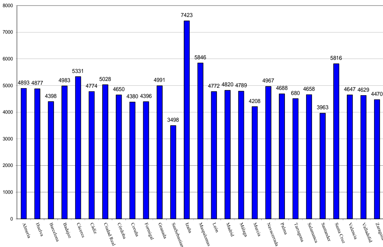
VALORES MEDIO DIARIOS DE RADIACIÓN UV Eritemática EN DISTINTAS ESTACIONES DE LA RED JULIO/2019(J/m 2 )
