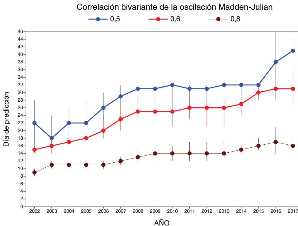
Figura 1. Evolución de los índices de acierto para la oscilación Madden-Julian desde 2002. Los índices de acierto se han calculado sobre la media de las retropredicciones del CEPMPM producidas durante un año completo. Las líneas azul, roja y marrón indican, respectivamente, el alcance de la predicción en días para el que la correlación bivalente de la citada oscilación toma los valores 0,5, 0,6 y 0,8. Esta gráfica muestra que los pronósticos de la oscilación Madden-Julian son significativamente más acertados ahora que hace 15 años (en 2017 la correlación 0,6 se alcanza el día 30 en lugar de alcanzarse el día 15, como ocurría en 2002).
