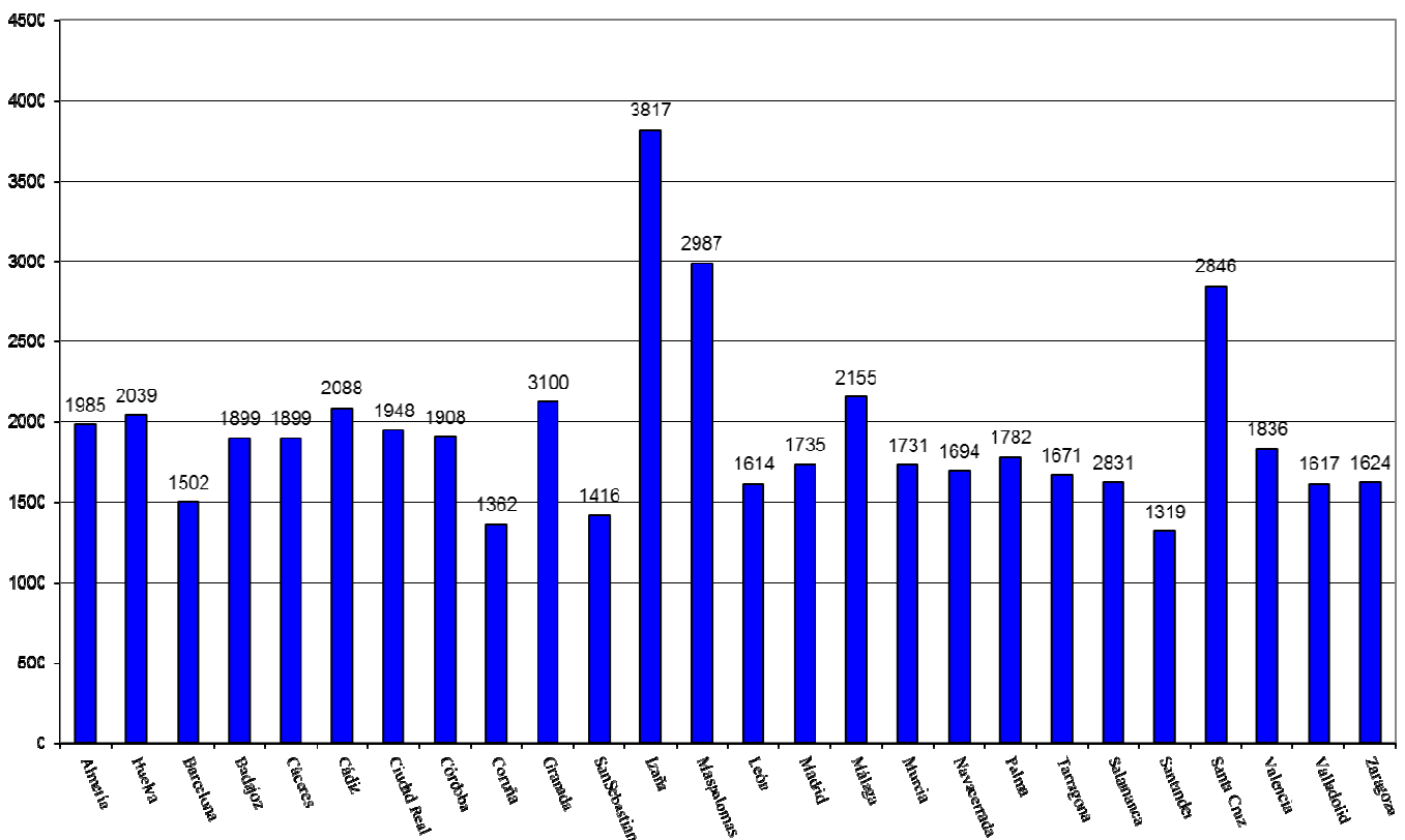
VALORES MEDIO DIARIOS DE RADIACIÓN UV Eritemática EN DISTINTAS ESTACIONES DE LA RED OCTUBRE/2019(J/m 2 )
