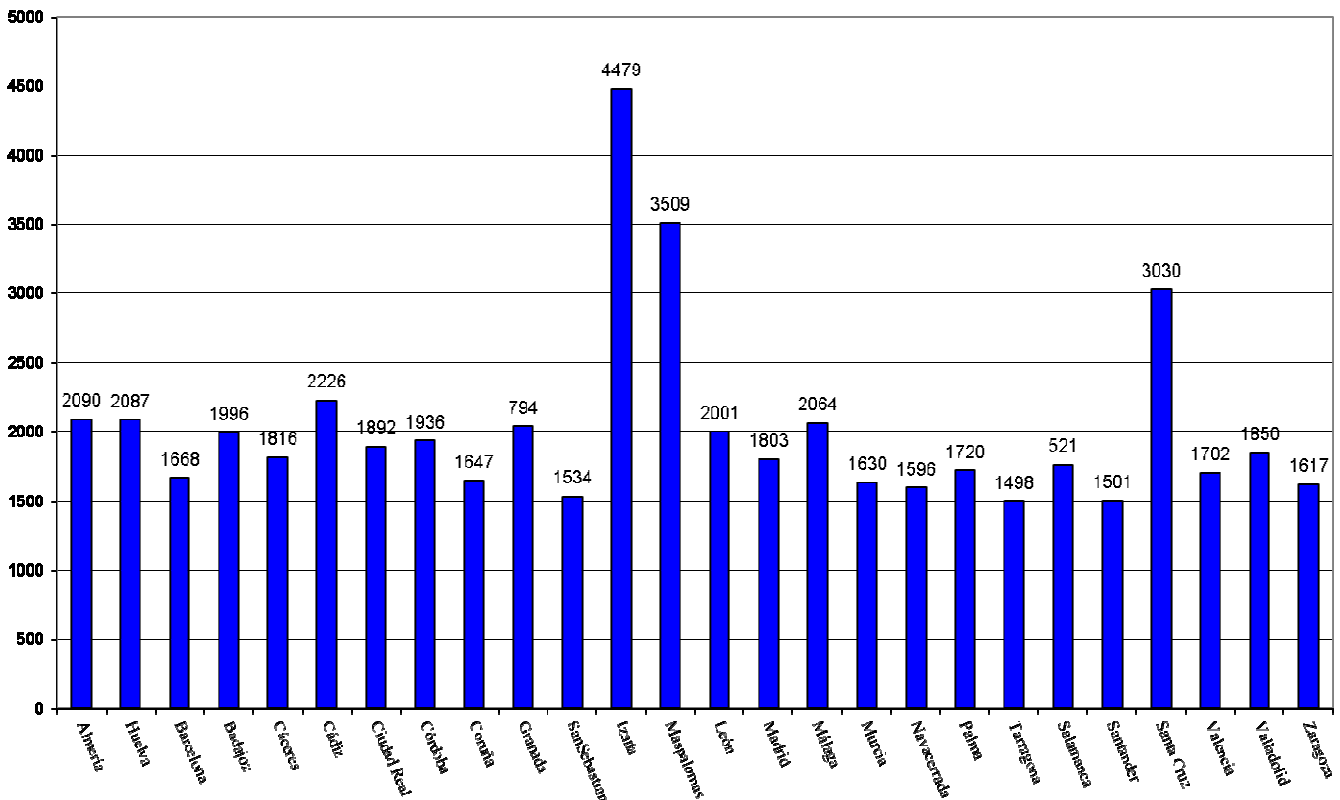
VALORES MEDIO DIARIOS DE RADIACIÓN UV Eritemática EN DISTINTAS ESTACIONES DE LA RED FEBRERO/2020(J/m 2 )
