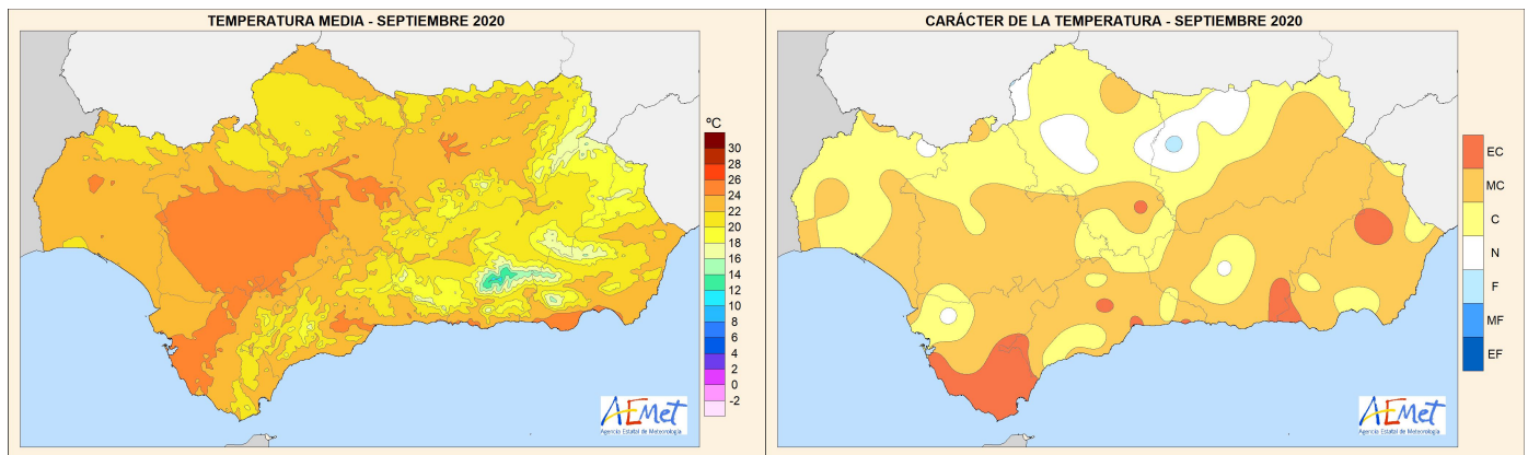
Temperatura media
