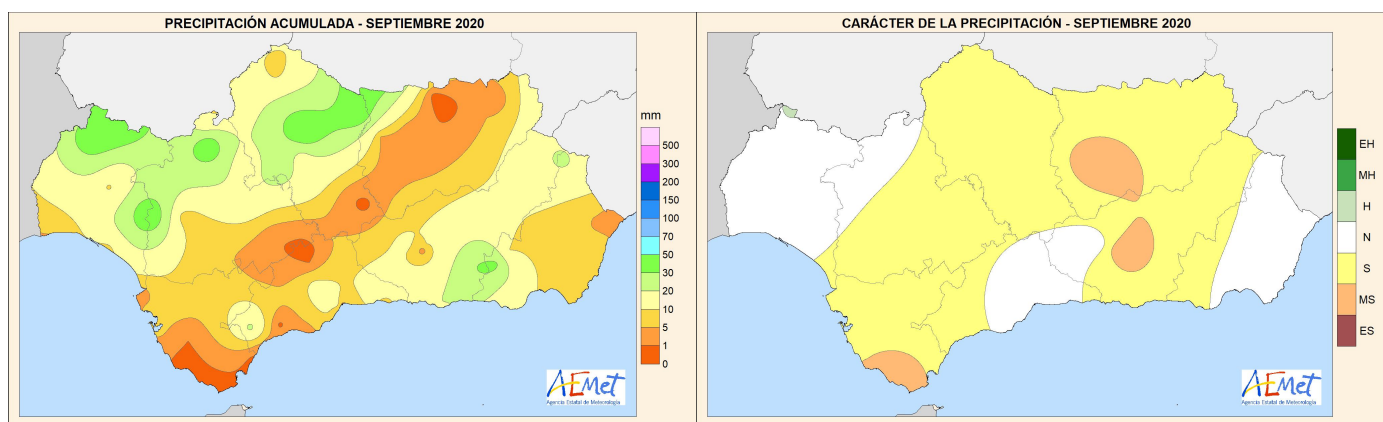
Precipitación mensual
