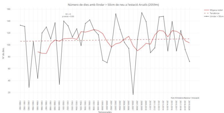
Fig. 3: GN50 umbral de espesor de nieve superior a 50cm en la estación de Arcalís a 2029m en las temporadas entre 1980 y 2020.
