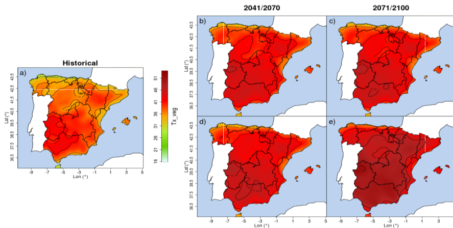
Fig.3. Representación geográfica de los valores esperados de temperatura máxima durante el periodo vegetativo (abril a octubre) para los periodos 2041-2070 y 2071-2100. Se representan ambos escenarios de emisiones: RCP4.5 (figuras b y c) y RCP8.5 (figuras d y e). La figura 5a representa los valores correspondientes al periodo Historical (1976-2005).
