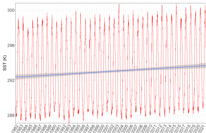
Fig. 3: Evolución temporal de la serie diaria de SST media del Mediterráneo (línea roja) y su tendencia lineal (línea azul) en el periodo 1982-2021.
