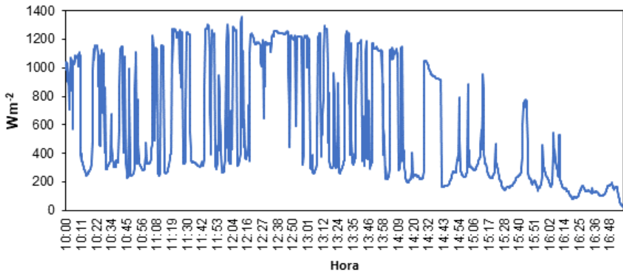
Fig. 3: Radiación de onda corta entrante ( S_{\downarrow} ) durante el 23 de febrero de 2018.
