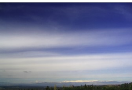
Altostratos
