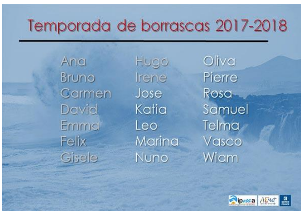
Nombres de las borrascas con gran impacto de la temporada 2017-2018
