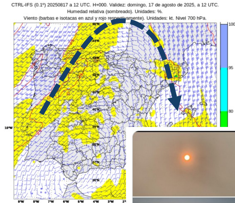
Viento en el nivel de 700 hPa
