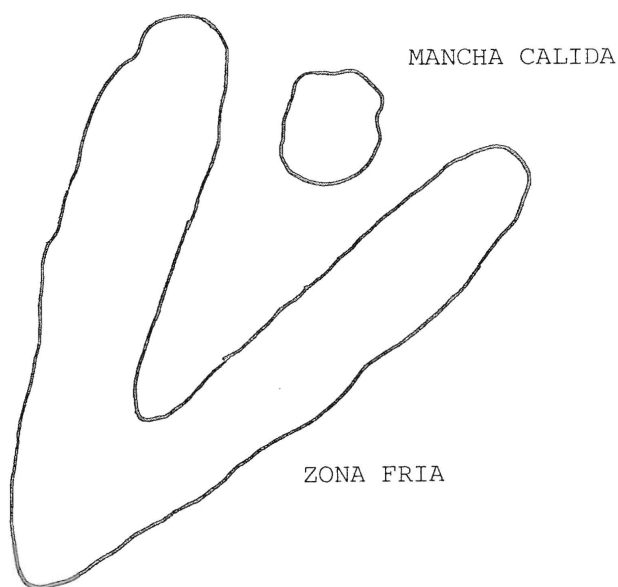
Figura 28.—Realce en "V" y mancha cálida (según McCann, 1981).
