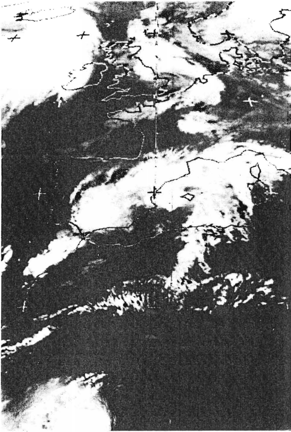
Figura 21.—METEOSAT IR: 15 de noviembre de 1985 a 12,00 TMG.
