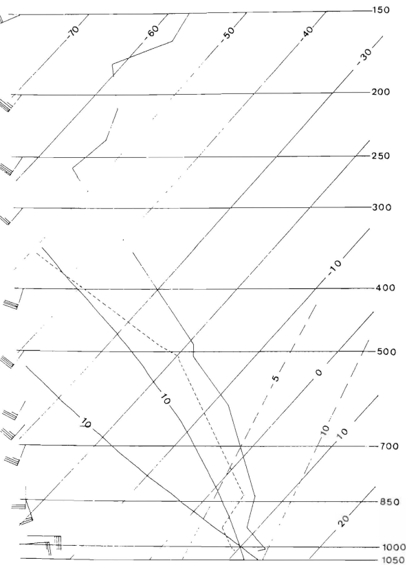
Figura 13.—Radiosondeo de Palma de Mallorca: 15 de noviembre de 1985 a 12 TMG.
