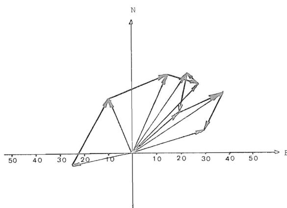
Figura 29.—Hodógrafa del viento en Palma de Mallorca el 15 de noviembre de 1985 a 12 TMG.
