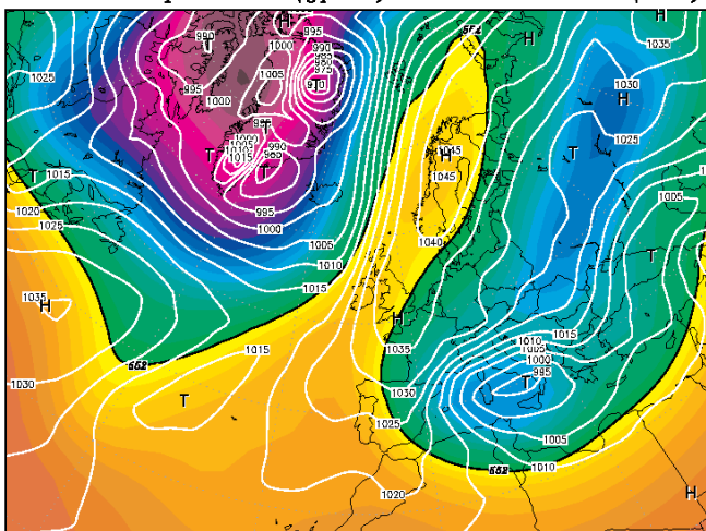
03FEB1956 00Z 500 hPa Geopotential (gpm) und Bodendruck (hPa)
