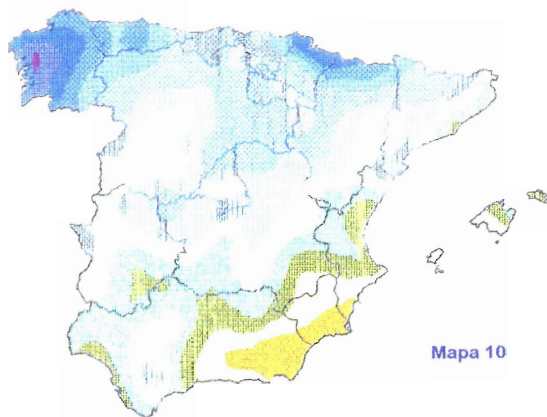
PRECIPITACIÓN ACUMULADA (mm) EN EL MES Abr. 99
