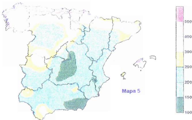
% HUMEDAD DEL SUELO / SATURACIÓN
