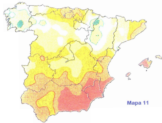
PORCENTAJE DE LA PREC. ACU. SOBRE LA NORMAL EN EL MES Abr. 99
