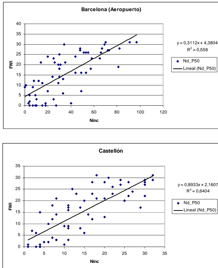
Fig.6. Valores medios mensuales de FWI frente al número mensual de incendios en las provincias de Barcelona y Castellón.
