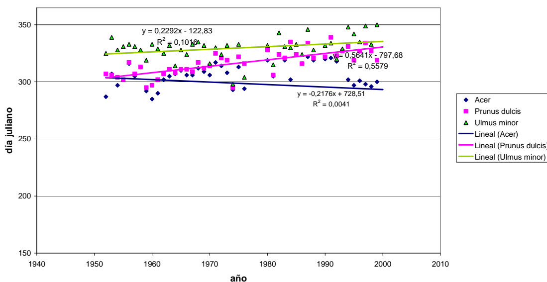
Fig.5. Series temporales de observaciones de la caída de la hoja de Arce, Olmo y Almendro con datos de la estación fenológica de Cardedeu (Barcelona).
