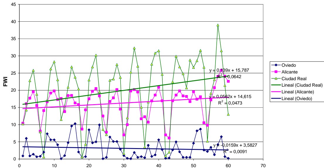
Evolución temporal del valor medio mensual del FWI en estaciones españolas (meses mayo-octubre de 1997-2006)
