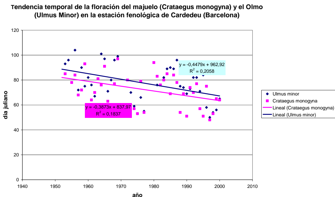
Fig. 4. Series temporales de observaciones de la floración de majuelo y Olmo con datos de la estación fenológica de Cardedeu (Barcelona).
