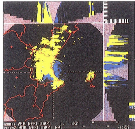
IMÁGENES: D11-2.a (superior-derecha); D11-2.b (centro-izquierda); D11-2.c (centro-derecha); D11-2.d (inferior-izquierda); D11-2.e (inferior-derecha) Análisis de ecos de tierra para el Radar de Valencia. (Explicación en el texto).
