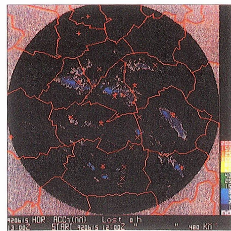
IMÁGENES: D11-1.a (superior-izquierda); D11-1.b (superior-derecha); D11-1.c (centro-izquierda); D11-1.d (centro-derecha); D11-1.e (inferior-izquierda); D11-1.f (inferior-derecha) Análisis de ecos de tierra para el Radar de Madrid. (Explicación en el texto).
