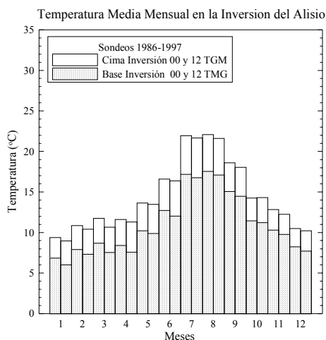
Figura 7: Temperatura media mensual en la inversión del Alisio a las 00 y 12 TMG.
