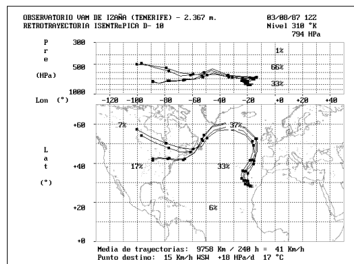
Figura 4: Ejemplo de una retro trayectoria isentrópica en IZO.
