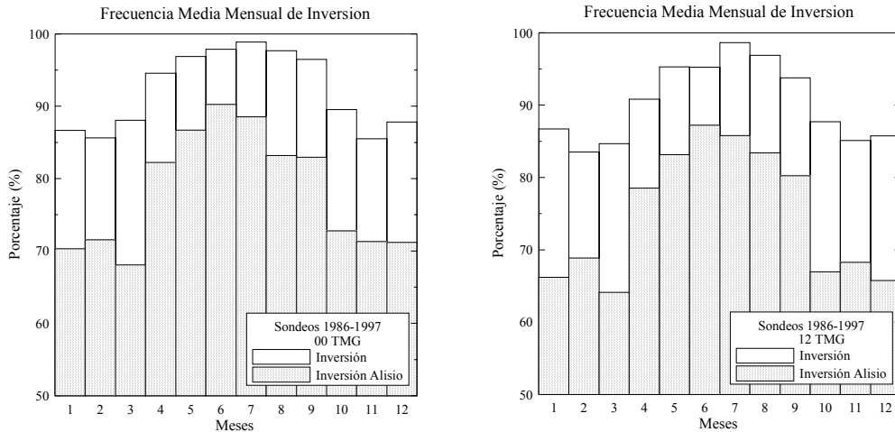
Figura 3: Frecuencia media mensual de inversión a las 00 TMG (izquierda) y 12 TMG (derecha).
