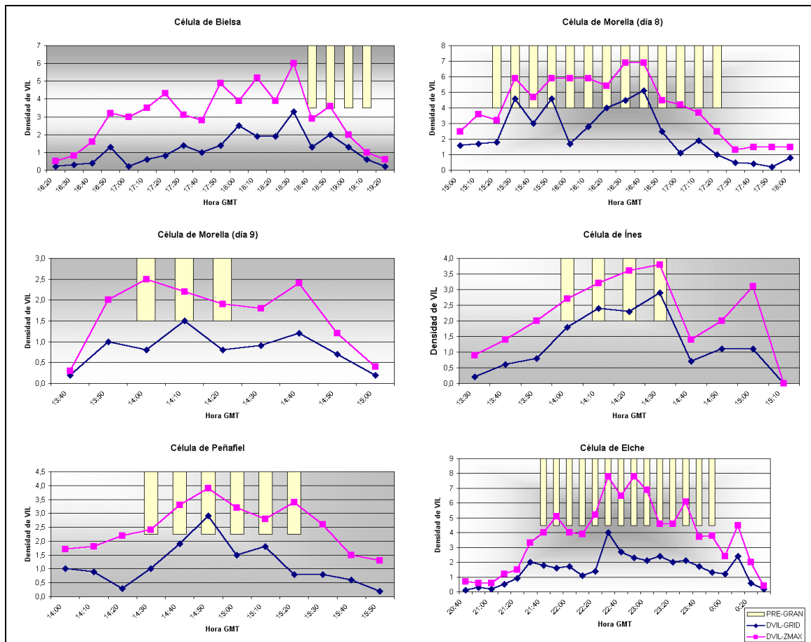
Figura 2: Evolución de las Densidades de VIL, DVIL-grid y DVIL-zmax, y precipitación con granizo.
