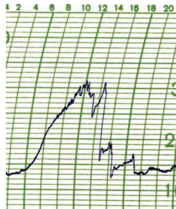
Extraordinario descenso térmico de más de 15\text{ }^{\circ}\text{C} en menos de 30 minutos durante la intensa tormenta del 23 de junio de 2006, día en el que varias trombas acumularon 52,2 mm de lluvia. Entre las 14,30 y las 15 horas (tiempo universal), la temperatura bajó de 31 a 16\text{ }^{\circ}\text{C} .
