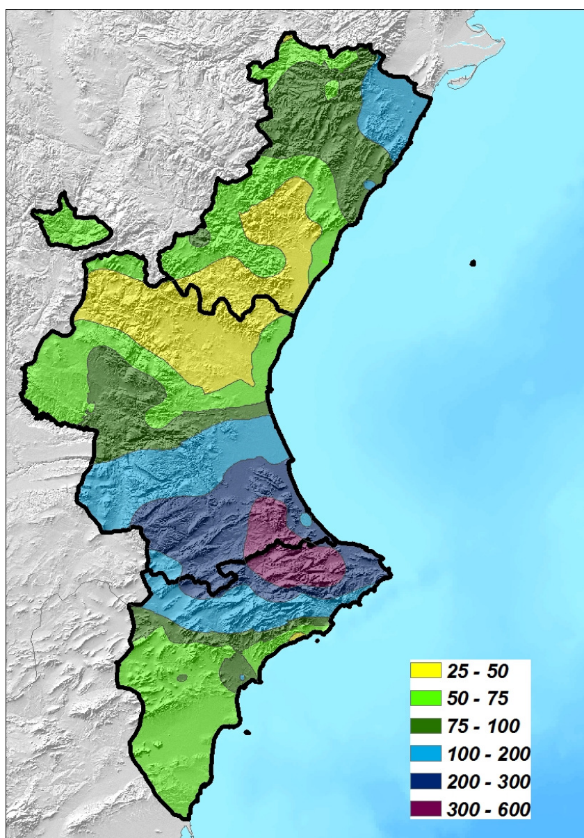
Figura 3 Precipitación acumulada en la Comunidad Valenciana en noviembre de 2012
