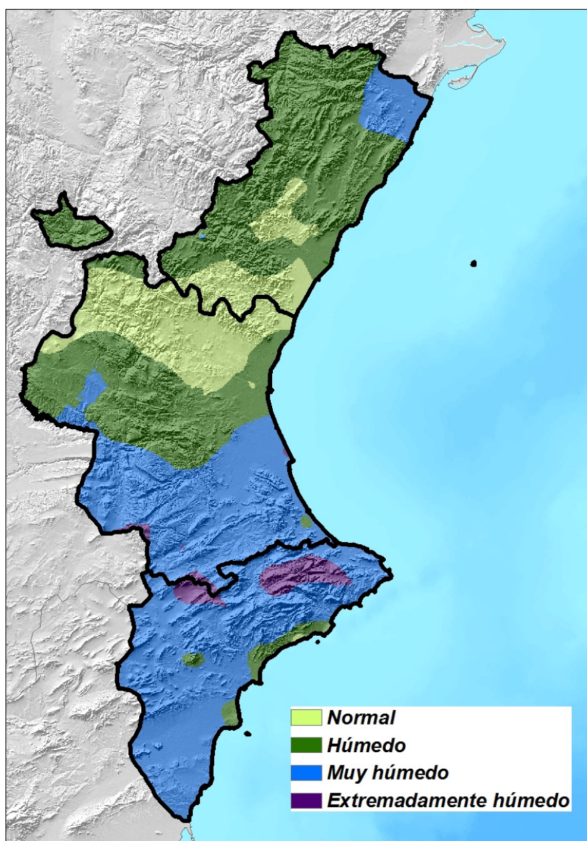
Figura 5 Calificación pluviométrica del mes de noviembre de 2012 en la Comunidad Valenciana
