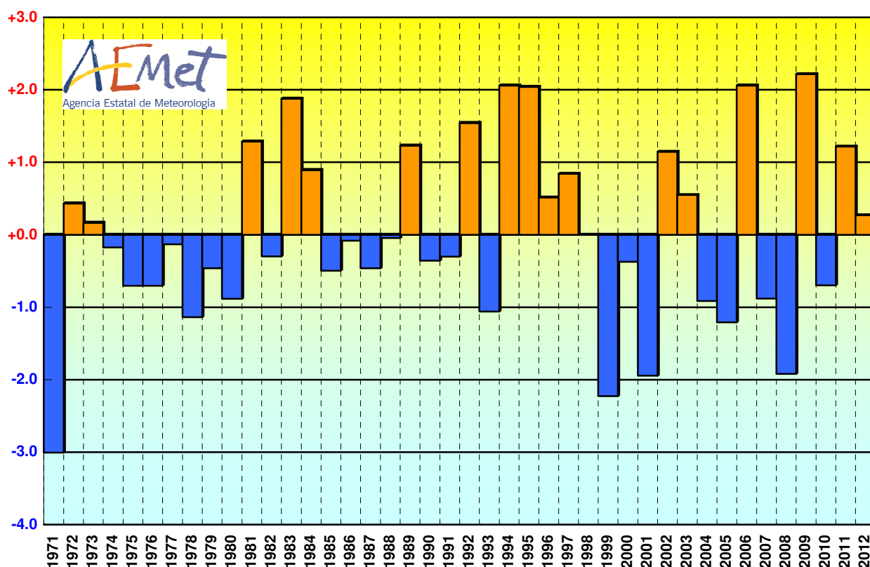
Figura 1 Anomalía de la temperatura media en la Comunidad Valenciana en noviembre (1971-2012)
