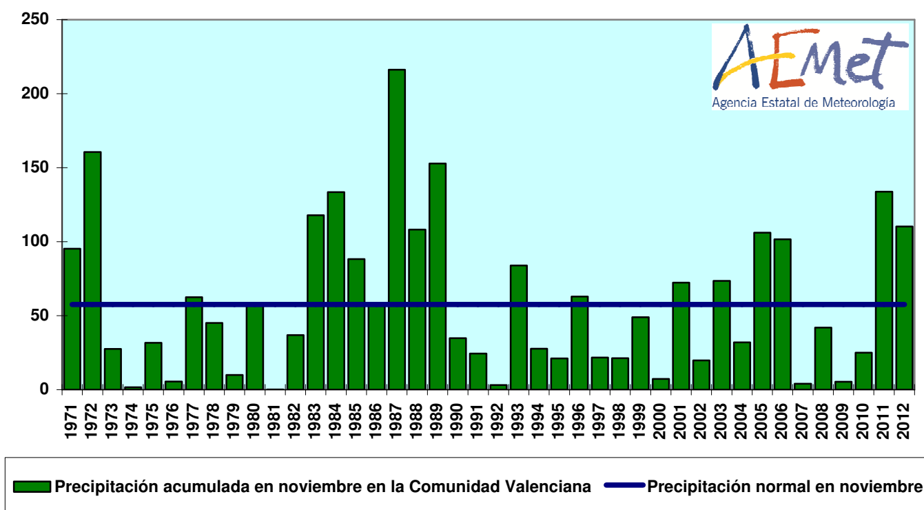
Figura 6 Evolución de la precipitación en la Comunidad Valenciana en noviembre (1971 a 2012)
