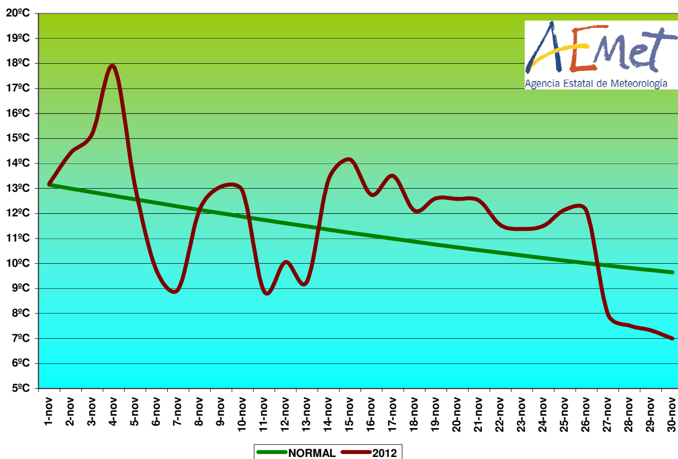
Figura 2 Temperatura media diaria estimada en la Comunidad Valenciana (noviembre de 2012 frente a lo normal)
