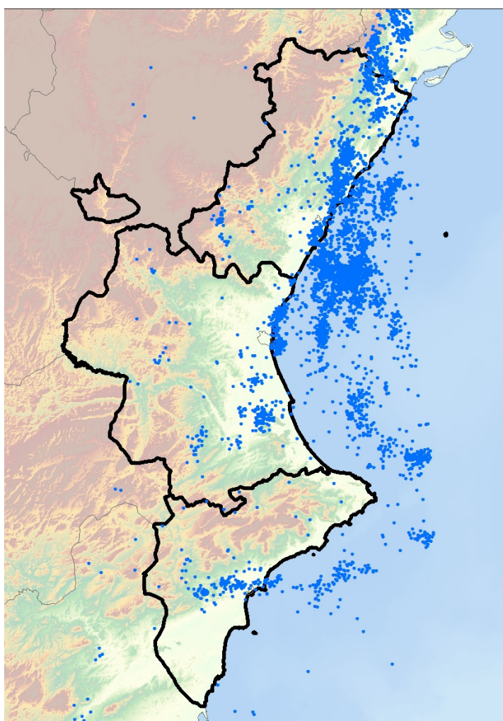
Figura 4 Rayos registrados en la Comunidad Valenciana (entre el mediodía del día 17 de noviembre y el mediodía del día 18 de noviembre de 2012).
