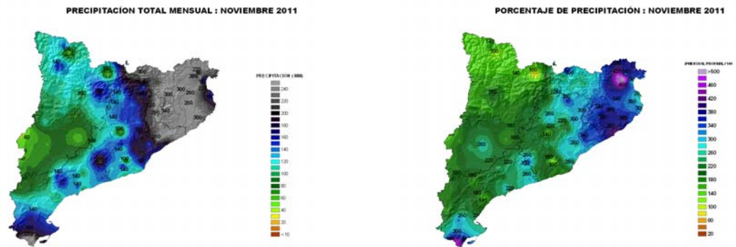
Precipitación acumulada y porcentaje
