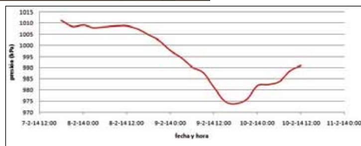
Figura 2: presión en el centro de la baja en superficie
