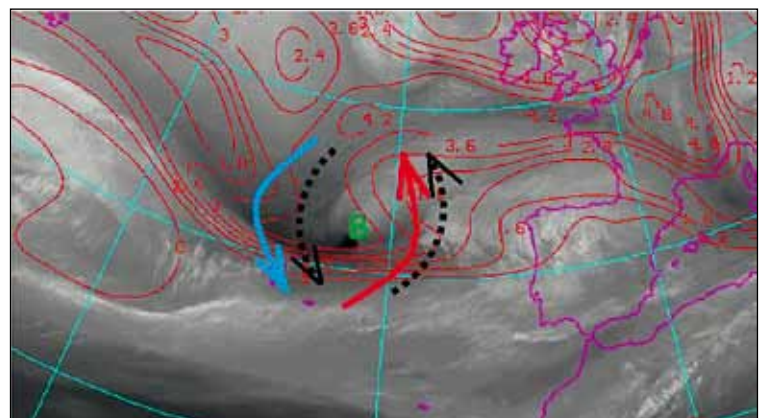
Figura 5: interacción entre la anomalía de niveles altos y la de niveles bajos superpuesta a la imagen de vapor de agua del domingo 9 a las 06 UTC y a los valores de vorticidad potencial (PV) en 300hPa (líneas rojas). (Fuente: Aemet)
