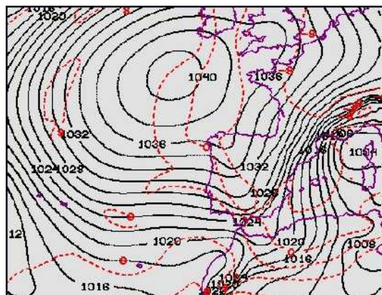
SITUACIÓN DEL DÍA 5 DE ENERO 2008, A 00 horas UTC: ARRIBA: ANALISIS EN 500 HPA; Altura geopotencial (negro) en intervalos de 60 msp, e isotermas (rojo) en intervalos de 4 °C. ABAJO: ANALISIS EN SUPERFICIE: Presión (negro) en intervalos de 2 Hpa, e isotermas en 850HPa en intervalos de 4 °C. (rojo).
