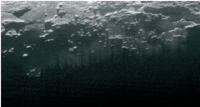
Figura 7. Nieblas a la puesta de Sol.
