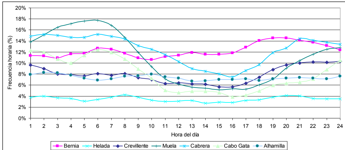
Fig. 5: Porcentaje de horas con recolección de niebla en función de la hora del día, durante el periodo comprendido entre enero de 2010 y abril de 2011
