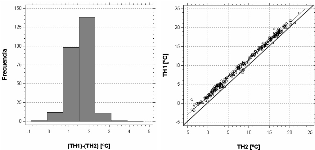
Fig. 2 (izquierda): Histograma de las diferencias de temperatura mínima del aire ( ^{\circ}\text{C} ) medida dentro (TH1) y fuera (TH2) de la garita meteorológica. Fig. 3 (derecha): Scatterplot de la temperatura mínima de aire medida en pareado dentro (TH1) y fuera (TH2) de la garita meteorológica. La bisectriz del cuadrante representa la recta de igual temperatura entre ambos sensores
