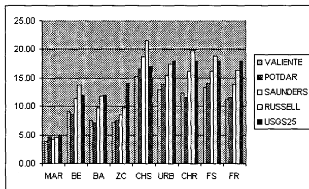
Fig. 4: Comparación de albedos para 9 clases del MUS'97. Clases: Agua marina (MAR), Urbano (URB), Cultivos herbáceos de secano (CHS), Cultivos herbáceos de regadío (CHR), Frutales de Secano (FS), Frutales de regadío (FR), Bosques de esclerófilas (BE), Bosques de aciculifolias (BA) y Zonas quemadas (ZC).
