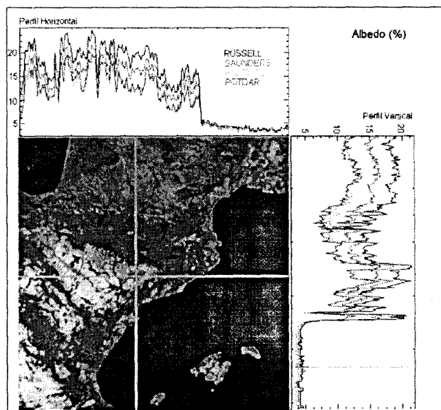
Fig. 6: Perfiles horizontal y vertical de los cuatro albedos calculados con AVHRR.
