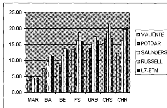
Fig. 5: Comparación de albedos AVHRR (cuatro autores) y albedo con LANDSAT.
