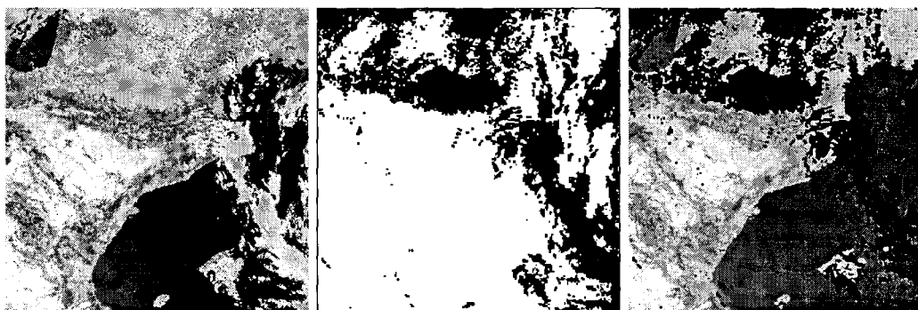
Fig. 2: Filtrado de nubes. RGB 3:2:1 de la imagen del día 4 de agosto de 1998 (Izq.), máscara de nubes (Centro) y RGB 3:2:1 sin nubes (derecha).
