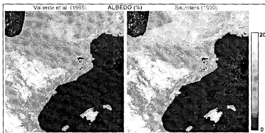
Fig. 3: Imágenes de albedo medio para el mes de agosto de 1998. Fórmulas de cálculo según VALIENTE et al. (1995) (Izq.) y según SAUNDERS (1990) (derecha).
