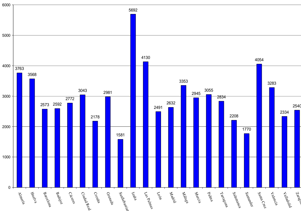
VALORES MEDIO DIARIOS DE LA RADIACIÓN UV-B EN DISTINTAS ESTACIONES DE LA RED ABRIL-2012 (J/m 2 )
