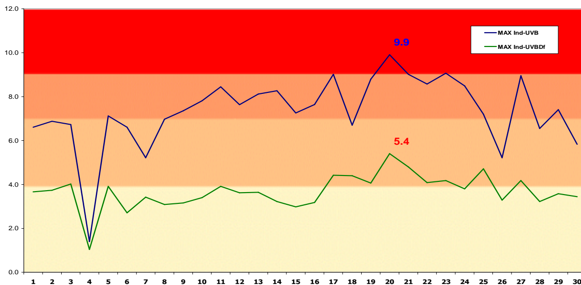
Evolución del Índice Máximo diario - UVB - UVB Difusa - MADRID ABRIL 2012
