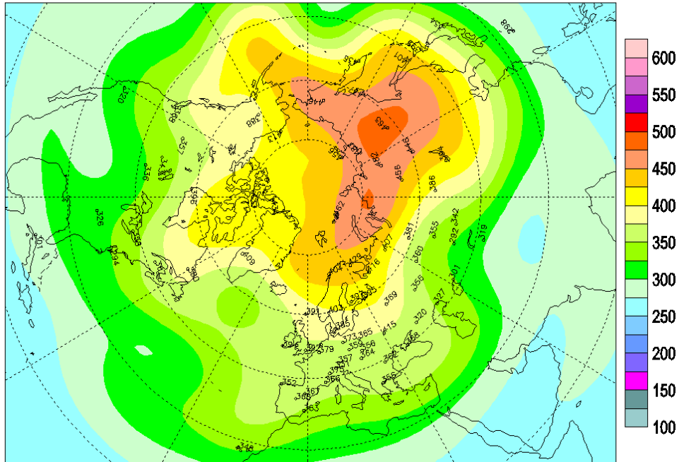
Mean total ozone (DU), 2012/04/01-2012/04/30
