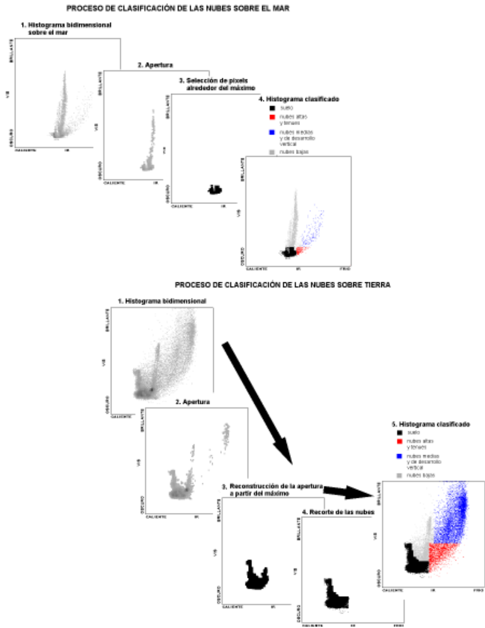
Figura 1. Proceso de clasificación morfológica de la nubosidad
