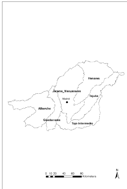
Figura 1: Cuencas hidrográficas seleccionadas
