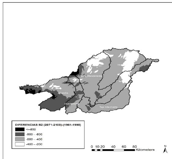
Figura 10: Diferencias entre la situación actual y el escenario B2
