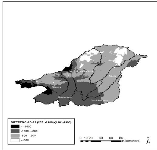
Figura 9: Diferencias entre la situación actual y el escenario A2
