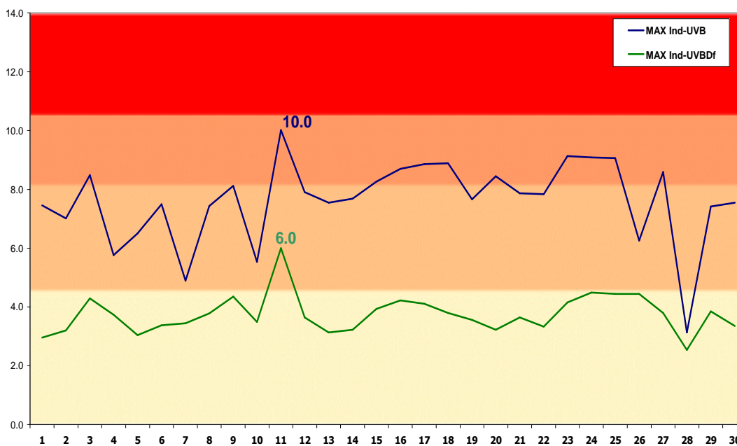
Evolución del Índice Máximo diario de Radiación UVB y UVB Difusa - MADRID ABRIL 2013
