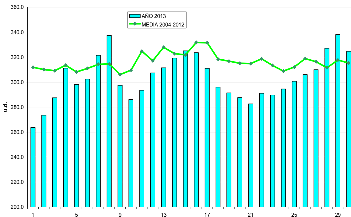
OZONO EN COLUMNA - SANTA CRUZ DE TENERIFE - ABRIL AÑO 2013
