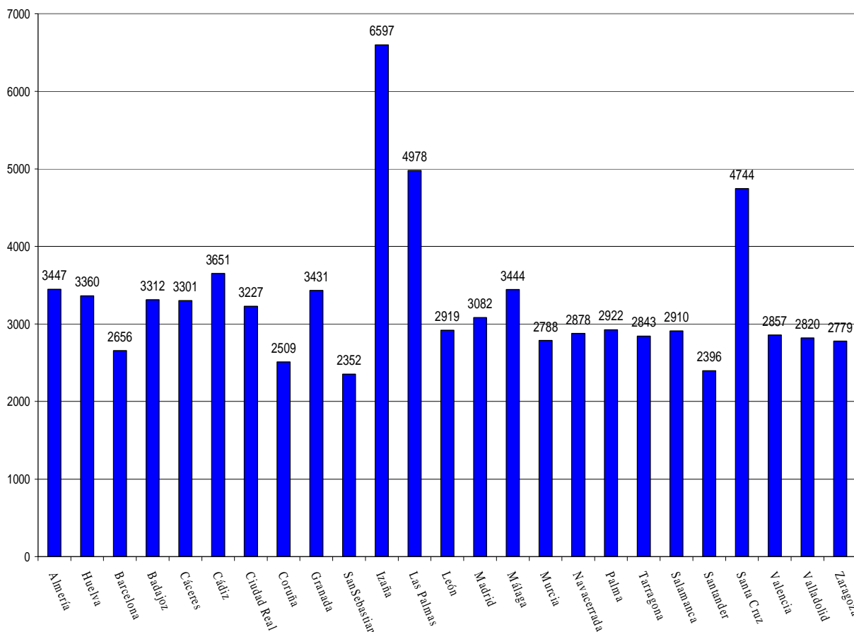
VALORES MEDIO DIARIOS DE LA RADIACIÓN UV-B EN DISTINTAS ESTACIONES DE LA RED ABRIL-2013 (J/m 2 )
