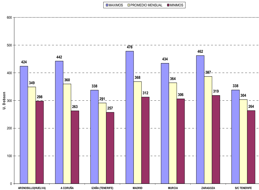
DATOS MENSUALES DE OZONO EN COLUMNA - ABRIL 2013
