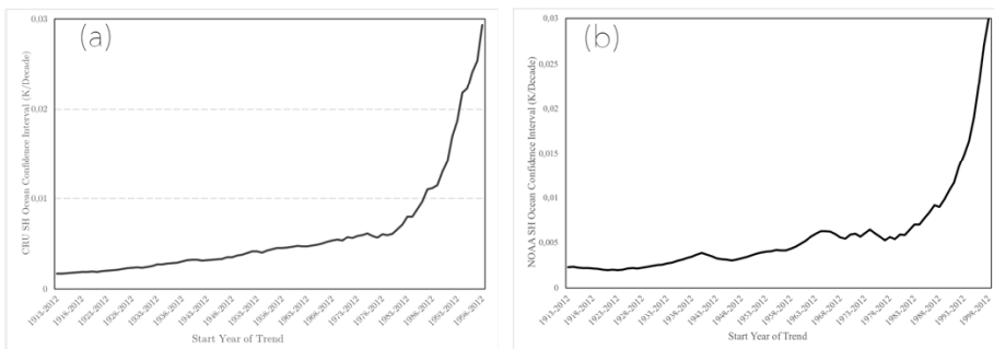
Figura 104: Evolución de los intervalos de confianza al 99% de la estimación de Sen de las diferentes bases de datos de hemisferio sur Ocean ventanas decrecientes entre 1913-2012 y 1998-2012 (es decir, en periodos entre 100 a 15 años). (a) CRU, (b) NOAA.
