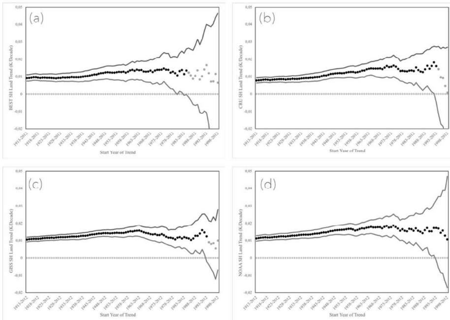
Figura 5: Estimación de tendencia (puntos negros) e intervalo de confianza al 99% (líneas sólidas) sobre las diferentes bases de datos de hemisferio sur Land con ventanas decrecientes entre 1913-2012 y 1998-2012 (es decir, en periodos entre 100 a 15 años). (a) BEST, (b) CRU, (c) GISS, y (d) NOAA. La significación estadística está identificada por la diferenciación de los puntos de color: negro: significativa ( p < 0.05 ); gris: no significativa ( p > 0.05 ) siguiendo los resultados de Mann Kendall.
