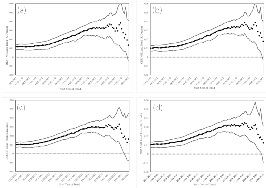
Figura 3: Estimación de tendencia (puntos negros) e intervalo de confianza al 99% (líneas sólidas) sobre las diferentes bases de datos de hemisferio norte Land con ventanas decrecientes entre 1913-2012 y 1998-2012 (es decir, en periodos entre 100 a 15 años). (a) BEST, (b) CRU, (c) GISS, y (d) NOAA. La significación estadística está identificada por la diferenciación de los puntos de color: negro: significativa ( p < 0.05 ); gris: no significativa ( p > 0.05 ) siguiendo los resultados de Mann Kendall.
