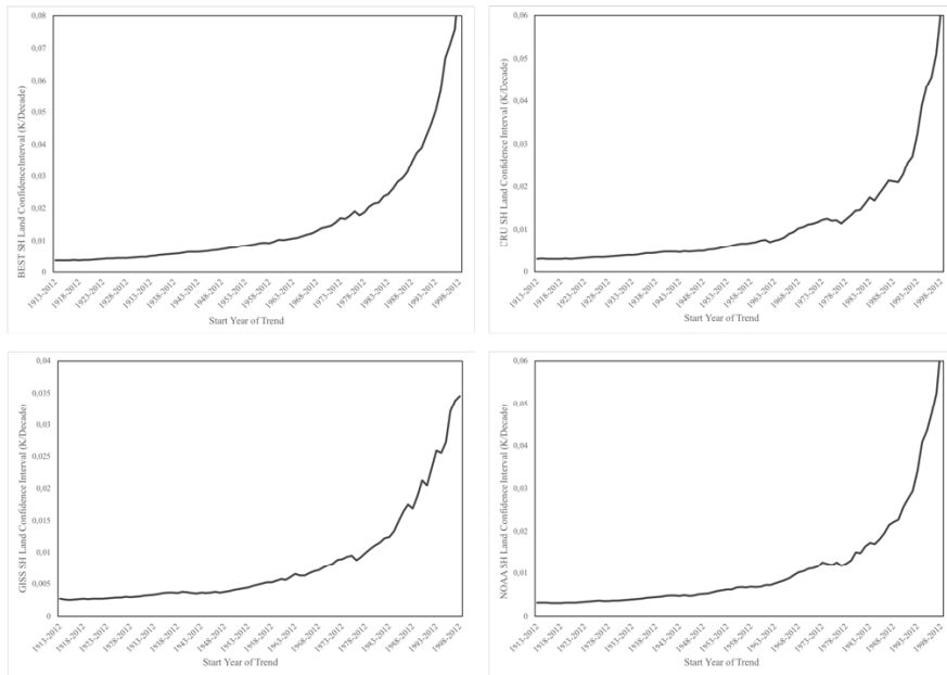
Figura 6: Evolución de los intervalos de confianza al 99% de la estimación de Sen de las diferentes bases de datos de hemisferio sur Land con ventanas decrecientes entre 1913-2012 y 1998-2012 (es decir, en periodos entre 100 a 15 años). (a) BEST, (b) CRU, (c) GISS, y (d) NOAA.
