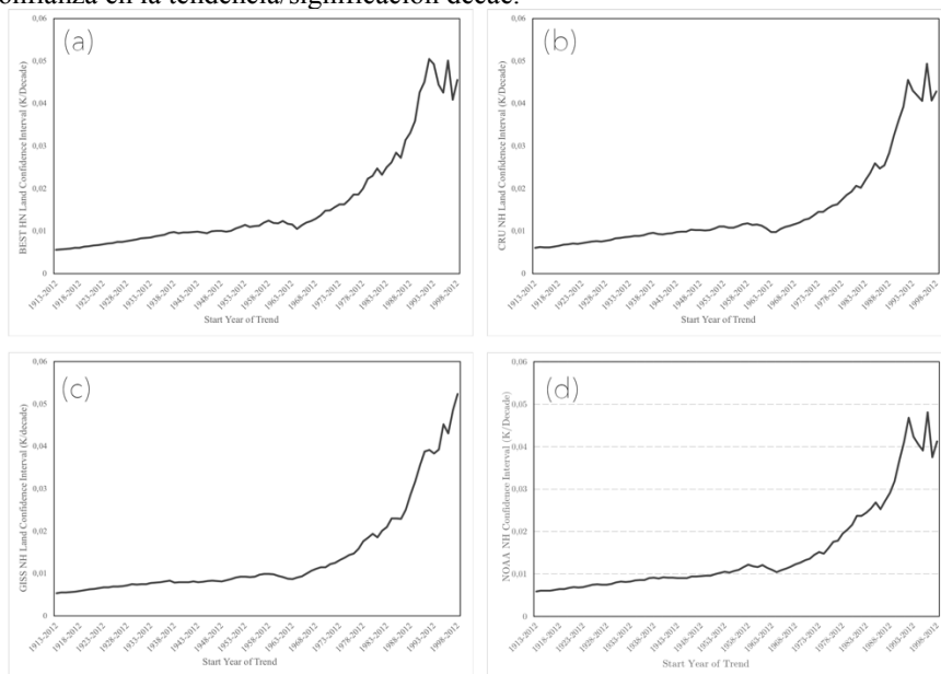
Figura 4: Evolución de los intervalos de confianza al 99% de la estimación de Sen de las diferentes bases de datos de hemisferio norte Land con una ventana de ventanas decrecientes entre 1913-2012 y 1998-2012 (es decir, en periodos entre 100 a 15 años). (a) BEST, (b) CRU, (c) GISS, y (d) NOAA.
