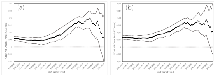
Figura 71: Estimación de tendencia (puntos negros) e intervalo de confianza al 99% (líneas sólidas) sobre las diferentes bases de datos de hemisferio norte Ocean con ventanas decrecientes entre 1913-2012 y 1998-2012 (es decir, en períodos entre 100 a 15 años). (a) CRU, (b) NOAA. La significación estadística está identificada por la diferenciación de los puntos de color: negro: significativa ( p < 0.05 ); gris: no significativa ( p > 0.05 ) siguiendo los resultados de Mann Kendall.
