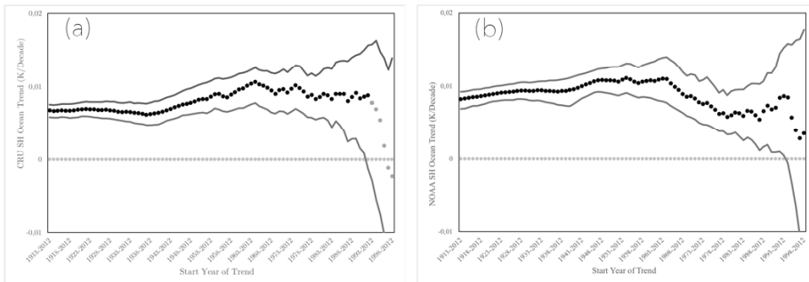
Figura 93: Estimación de tendencia (puntos negros) e intervalo de confianza al 99% (líneas sólidas) sobre las diferentes bases de datos de hemisferio sur Ocean ventanas decrecientes entre 1913-2012 y 1998-2012 (es decir, en periodos entre 100 a 15 años). (a) CRU, (b) NOAA. La significación estadística está identificada por la diferenciación de los puntos de color: negro: significativa ( p < 0.05 ); gris: no significativa ( p > 0.05 ) siguiendo los resultados de Mann Kendall.
