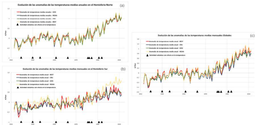
Figura 2: Valores de T_{mean} anual (1913-2012). Anomalías con base 1951-1980 (excepto NOAA 1901-2000). (a) hemisferio norte, (b) hemisferio sur y (c) Global.
