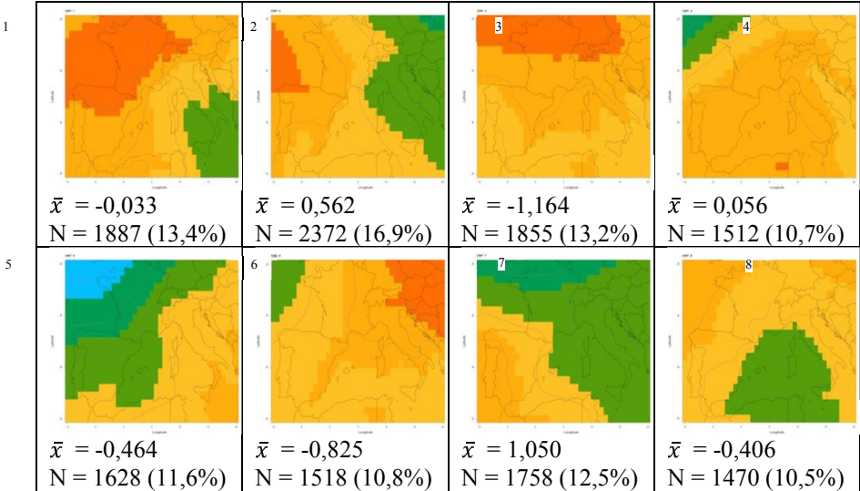
Fig. 8: Ídem Figura 2, para la ventana sinóptica 35°N–50°N y 10°O–20°E.
