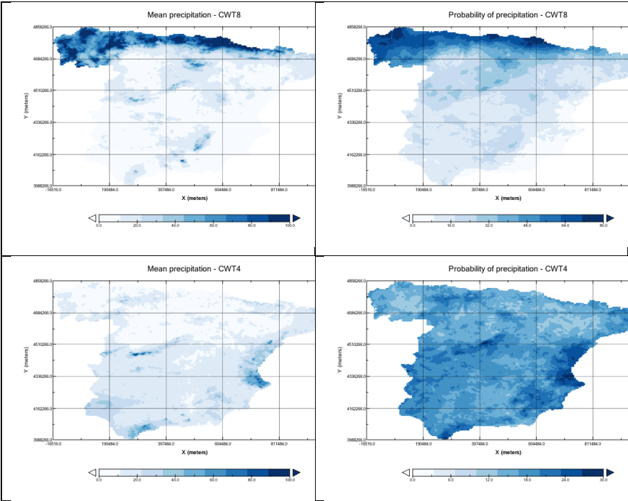
Fig. 5: Ídem Figura 3, para la ventana sinóptica 30°N–60°N y 15°O–20°E.
