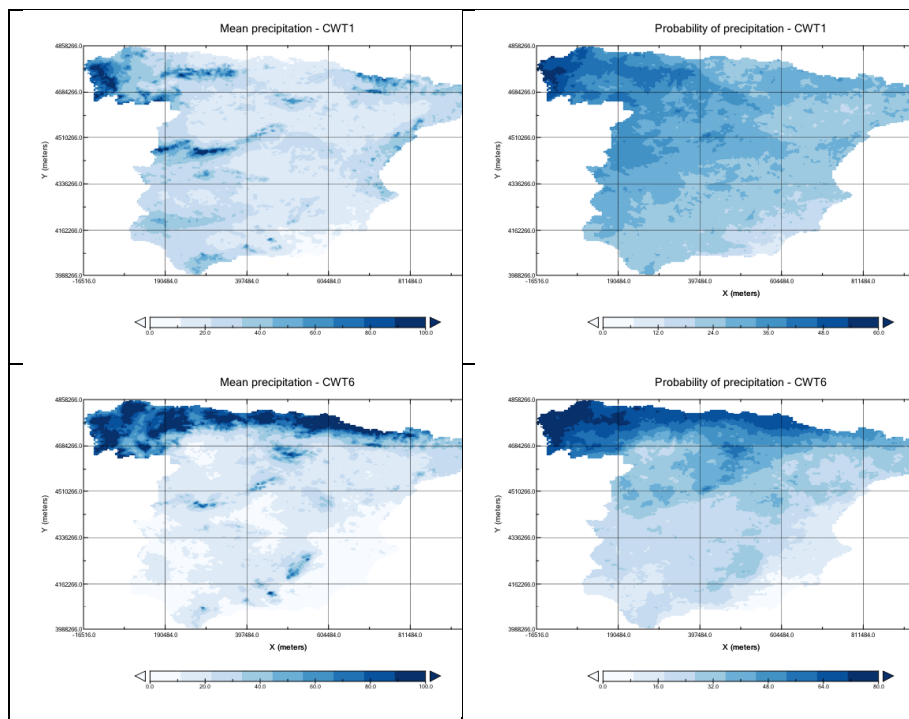
Fig. 11: Ídem Figura 3, para la ventana sinóptica 35°N–45°N y 10°W–15°E.
