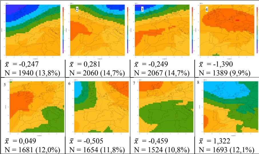
Fig. 4: Ídem Figura 2, para la ventana sinóptica 30°N–60°N y 15°O–20°E.
