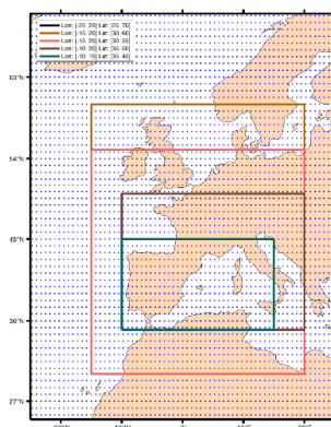
Fig. 1: Ventanas sinópticas de estudio. Fuente: elaboración propia.
