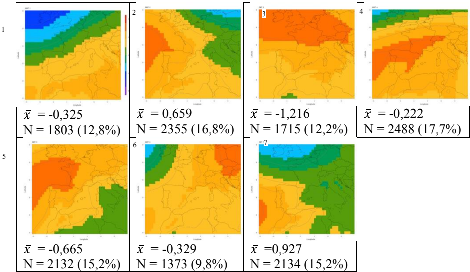
Fig. 6: Ídem Figura 2, para la ventana sinóptica 30°N–55°N y 15°W–20°E.
