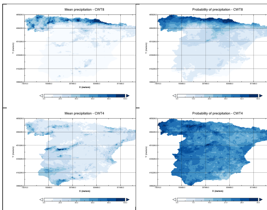
Fig. 3: Precipitación media (izq) y probabilidad de precipitación (dcha) de la España peninsular según el tipo 8 (fase positiva) (arriba) y el tipo 4 (fase negativa)
