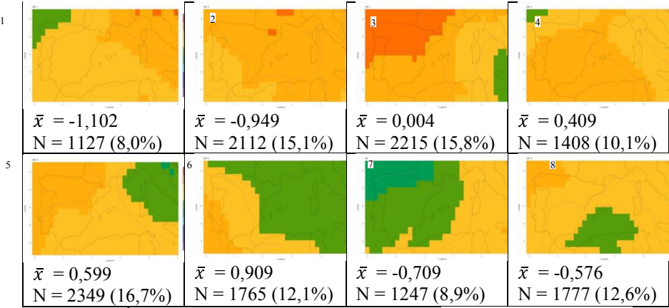
Fig. 10: Ídem Figura 2, para la ventana sinóptica 35°N–45°N y 10°W–15°E.
