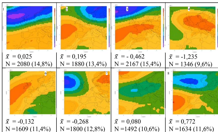
Fig. 2: Clasificación sinóptica en superficie, mediante COST733class, de la ventana sinóptica 25°N–70°N y 25°O–25°E, donde \bar{x} es el valor medio del WeMO instrumental y N el número de días incluidos en cada patrón de circulación atmosférica junto a su porcentaje respecto al total de días. Fuente: elaboración propia.
