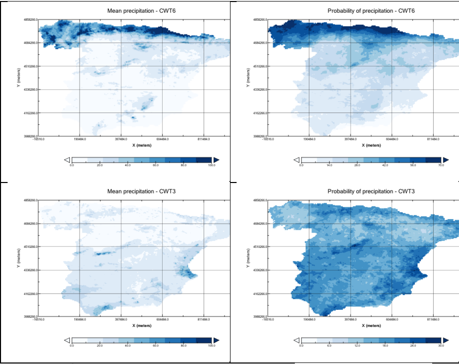
Fig. 7: Ídem Figura 3, para la ventana sinóptica 30°N–55°N y 15°O–20°E.
