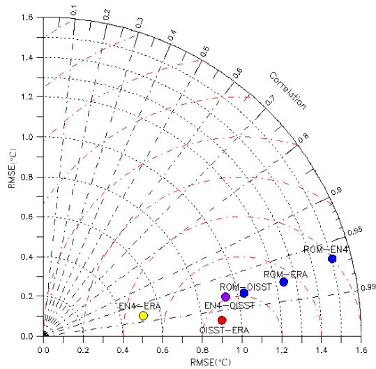
Fig. 4. Diagrama de Taylor de SST para el Mediterráneo durante 1980-2012. El diagrama resume la relación entre R^2 y RMSE ( ^{\circ}\text{C} ) para todas las comparaciones.
