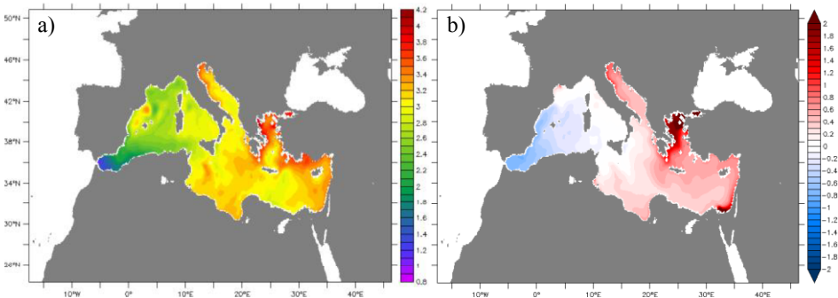
Fig.6. Distribución de la a) \Delta SST ( ^{\circ} C), b) \Delta SSS (psu) promedio establecido entre los periodos 2069-2099 y 1950-1980 en el Mar Mediterráneo.
