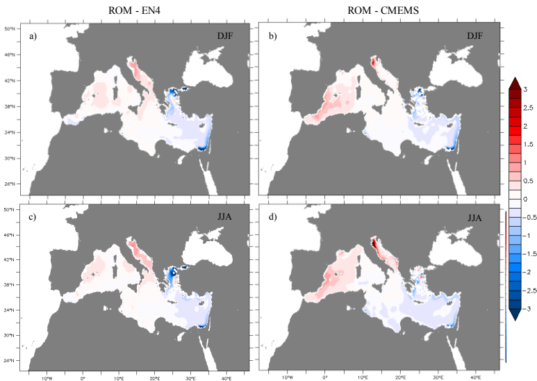
Fig. 5. Diferencias promedio de SSS (psu) entre ROM y distintas climatologías para los meses de invierno (DJF, panel superior) y verano (JJA, panel inferior)
