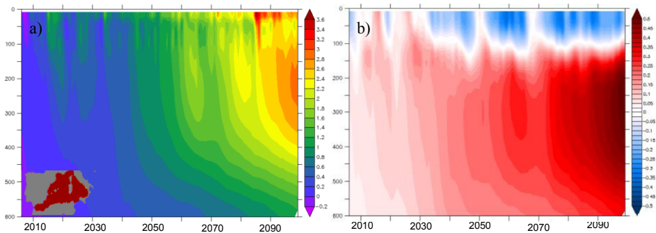
Fig. 7. Evolución temporal a lo largo de la columna de agua (600) m en la cuenca occidental; a) temperatura ( ^{\circ}\text{C} ); b) salinidad (psu).
