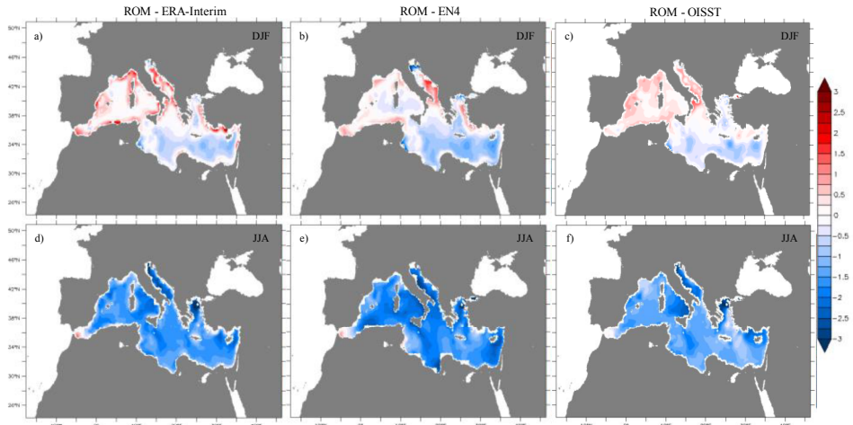
Fig. 3. Diferencias promedio de SST (°C) entre ROM y distintas climatologías para los meses de invierno (DJF, panel superior) y verano (JJA, panel inferior).
