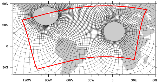
Fig. 2. Malla oceánica y atmosférica de ROM. Malla de resolución variable MPIOM (líneas negras, se dibuja cada duodécima), dominio REMO (línea roja).
