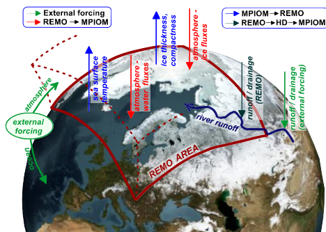
Fig. 1. Esquema de acoplamiento de ROM. Fuente: Cabos Narvaez et al. , 2014.
